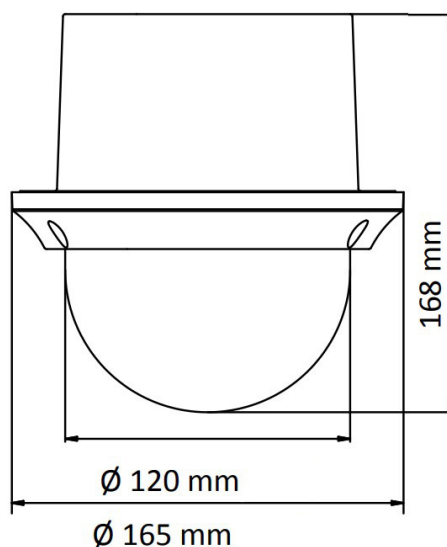
吸頂式安裝
